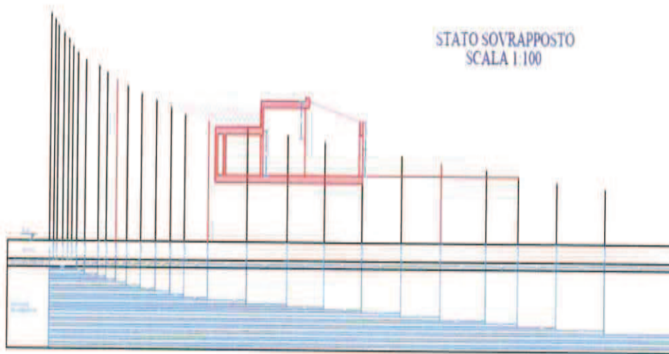
SEZ. B-B'
